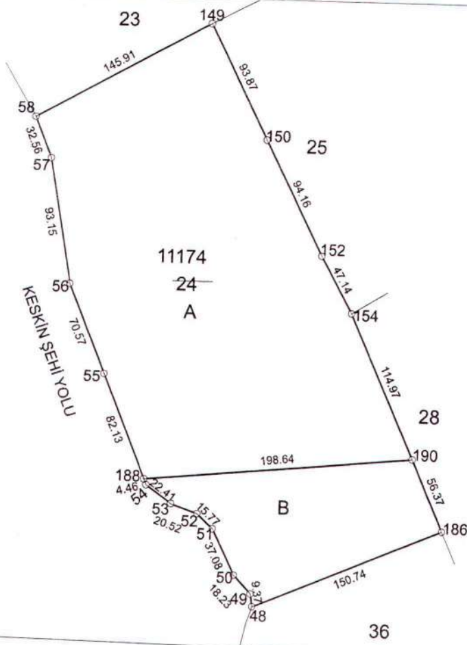
Poligon ve Köşe Koordinatları, Açık-Mesafe Bilgileri
