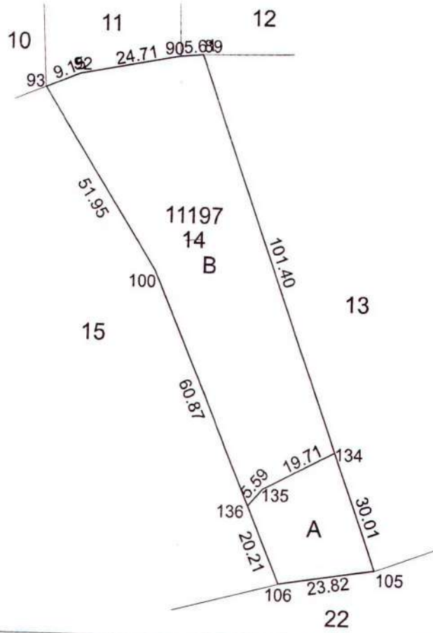
Poligon ve Köşe Koordinatları, Açılı-Mesafe Bilgileri
