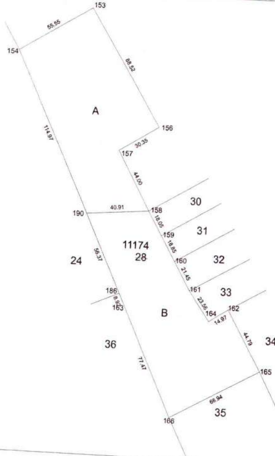
Poligon ve Köşe Koordinatları, Açı-Mesafe Bilgiler
