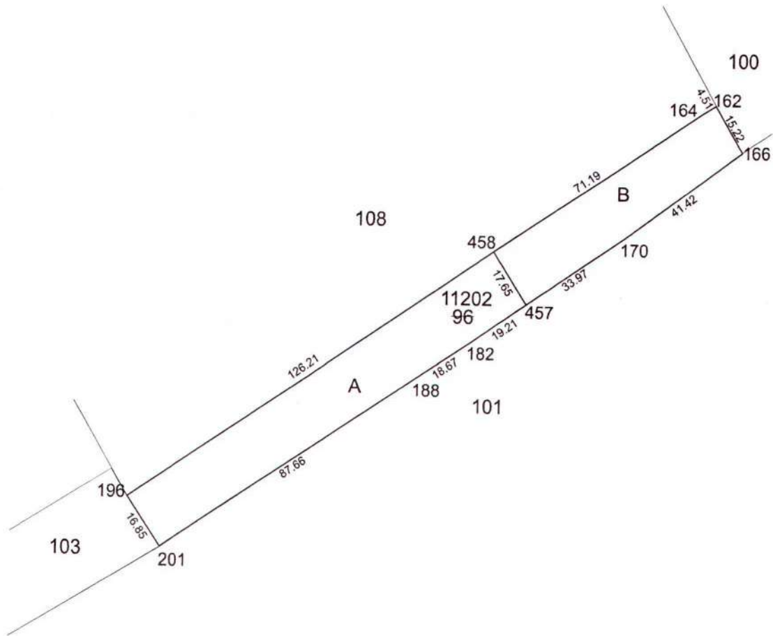
Poligon ve Köşe Koordinatları, Açı-Mesafe Bilgiler
