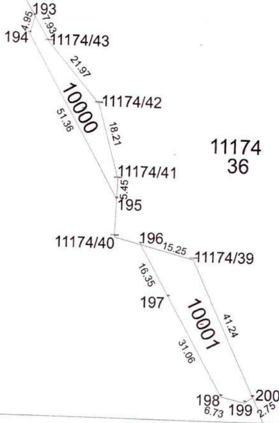
Poligon ve Köşe Koordinatları, Açılı-Mesafe Bilgileri
