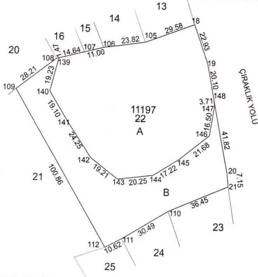
Poligon ve Köşe Koordinatları, Açılı-Mesafe Bilgileri
